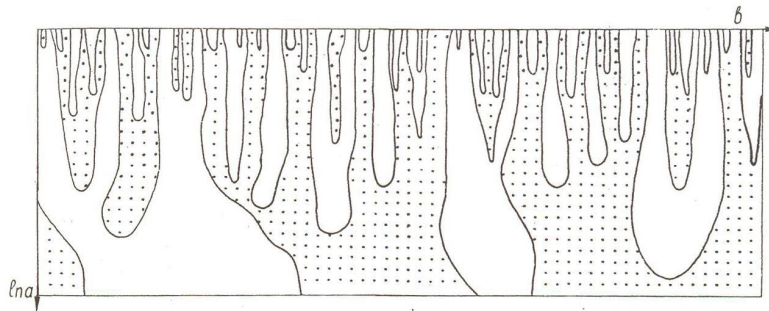
Рис. 1. Вейвлетное преобразование временного ряда ежедневных значений индекса зональной циркуляции атмосферы северного полушария Земли за пять месяцев в диапазоне от 1 до примерно 30 дней (вейвлетная функция - вещественная "мексиканская шляпа")
