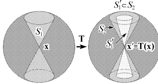
Рис. 5. К пояснению смысла условия для расширяющихся конусов S . Чтобы не загромождать рисунок, использована упрощенная версия обозначений: S_1 = S_x^\gamma , S_1' = \mathbf{DT}_x S_x^\gamma , S_2 = S_{\mathbf{T}(\mathbf{x})}^\gamma
