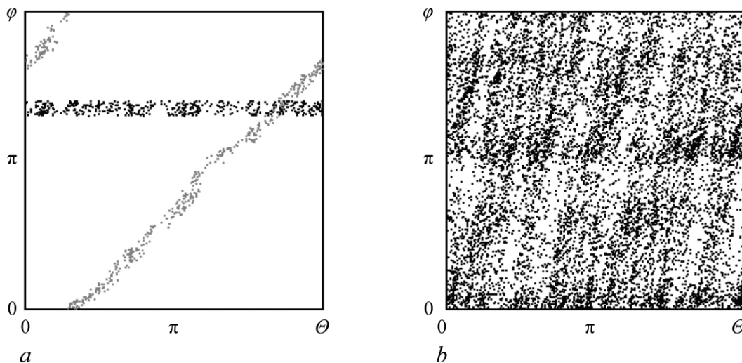
Рис. 5. Диаграмма, иллюстрирующая основное топологическое свойство стробоскопического отображения для фаз ( a ), и диаграмма, визуализирующая характерное для аттрактора Ханта–Отта распределение плотности вероятности на плоскости фазовых переменных ( b ). Диаграммы построены путем обработки временных рядов, полученных при моделировании динамики схемы в среде Multisim
