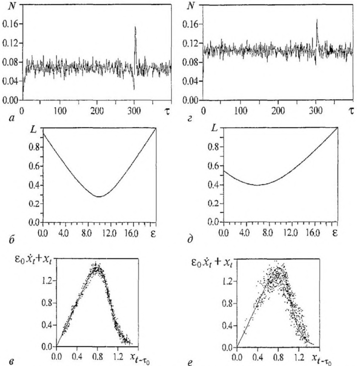
Рис. 5. Оценка времени запаздывания, параметра инерционности и восстановление функции по временным рядам уравнения Маккея - Гласса с добавленным гауссовым белым шумом. а, z - Нормированное число N пар экстремумов временного ряда, удаленных на \tau друг от друга, при 3% (а) и 10% (z) шуме. N(\tau) нормировано на общее число экстремумов временного ряда. N_{\min}(\tau)=N(300)=0.02 (а), N_{\min}(\tau)=N(300)=0.07 (z). б, д - Зависимость длины линии L , соединяющей последовательно точки на плоскости (x_{t-\tau_0}, \epsilon \dot{x}_t + x_t) , от \epsilon при 3% и 10% шуме, соответственно. L_{\min}(\epsilon)=L(9.9)=0.28 (б), L_{\min}(\epsilon)=L(6.0)=0.39 (д). в, е - Нелинейная функция (7) (сплошная линия) и восстановленная функция (точки) при 3% (в) и 10% (е) шуме и \epsilon , соответствующем минимуму L(\epsilon)
