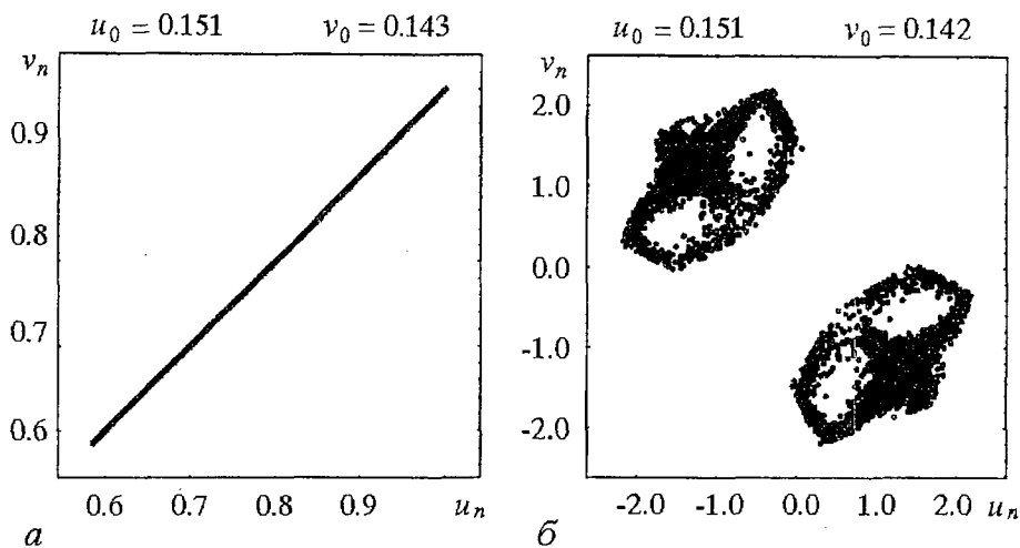
Рис. 5. Аттрактор системы двух связанных отображений (13) при \epsilon_i=0.433 , \epsilon_d=1.050 (режим слабой устойчивости). При построении диаграмм (а) и (б) выбраны разные стартовые точки ( u_0, v_0 )
