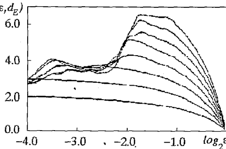
Рис.10. Дифференциальная размерность \tilde{D}_2^s(\varepsilon, d_E) для шума, равномерно распределенного в интервале [0,1] ; d_E изменяется от 2 до 10
