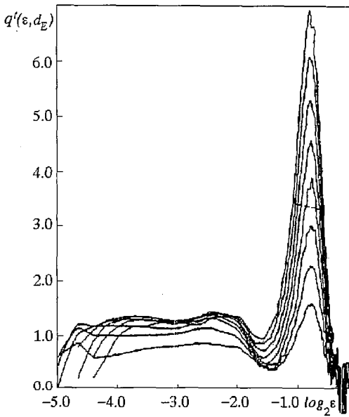
Рис. 9. Квадратичная компонента временного корреляционного интеграла q'(\epsilon, d_E) = \partial \tilde{D}_2'(\epsilon, d_E) / \partial \log \epsilon , d_E изменяется от 2 до 10
