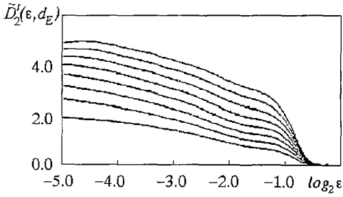
Рис. 7. Дифференциальная размерность \tilde{D}_2'(\epsilon, d_E) для временной наблюдаемой из рис. 3; d_E изменяется от 2 до 10
