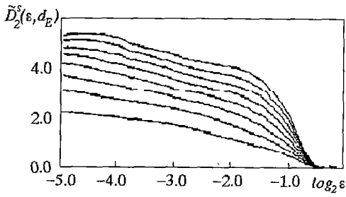
Рис. 4. Дифференциальная размерность \tilde{D}_2^s , вычисленная для пространственного распределения поля, взятого в один момент времени из стационарного пространственно-временного хаоса, изображенного на рис. 3; d_E изменяется от 2 до 10
