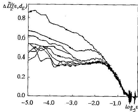
Рис. 5. \Delta \tilde{D}_2^s(\epsilon, d_E) = \tilde{D}_2^s(\epsilon, d_E) - \tilde{D}_2^s(\epsilon, d_E - 1) . Насыщение на графике при увеличении d_E от 2 до 9 происходит на уровне \Delta \tilde{D}_2^s(\epsilon, d_E) = 0.35
