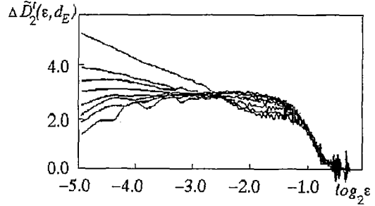
Рис. 8. Зависимость \sigma_2(\epsilon, d_E)t = \Delta \tilde{D}_2'(\epsilon, d_E) = \tilde{D}_2'(\epsilon, d_E) - \tilde{D}_2'(\epsilon, d_E - 1) . Насыщение на графике при увеличении d_E от 2 до 9 происходит на уровне \sigma_2 t = 0.33
