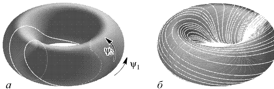
Рис. 6. Траектории на «фазовом торе»: a – резонансный двухчастотный тор с числом вращения w = 1/2 , b – трехчастотный тор. Параметры соответствуют рис. 3, d и e
